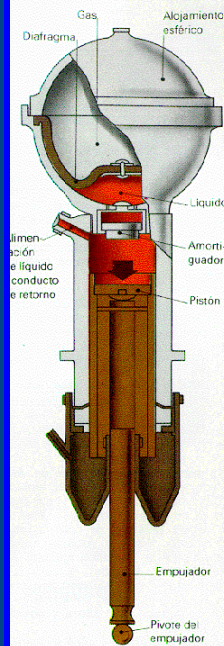
Sección transversal de la unidad de suspensión hidroneumática.
